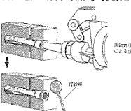
図 注入口付アンカーピンへのエポキシ樹脂の充填（引用：参考文献③）
