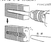
図 穿孔・清掃（引用：参考文献③）
