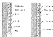
補修前 補修後 タイル張替え工法例(chord作成)
