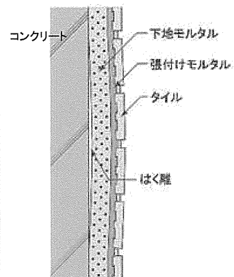
コンクリート・下地モルタル間のはく離
