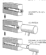
図 注入口付アンカーピンの打込み（引用：参考文献③）
